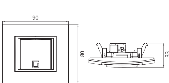
Switch Technical Drawings Desene Tehnice Întrerupător
