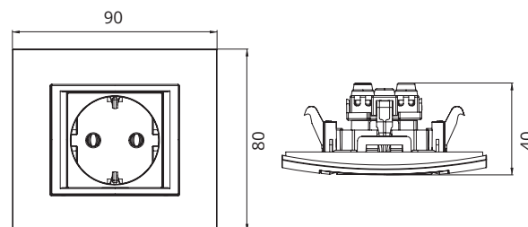
Socket Outlet Earthed Technical Drawings Desene Tehnice Priză Cu CP
