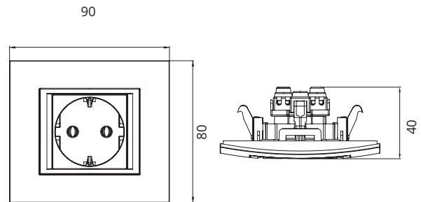
Socket Outlet Earthed Technical Drawings Desene Tehnice Priză Cu CP
