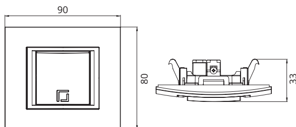
Switch Technical Drawing Desene Tehnice Întrerupător
