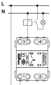
Кнопочный выключатель
