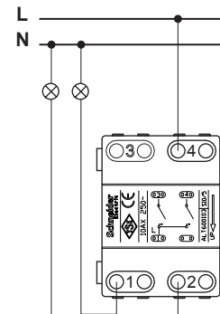
Двухклавишный выключатель
