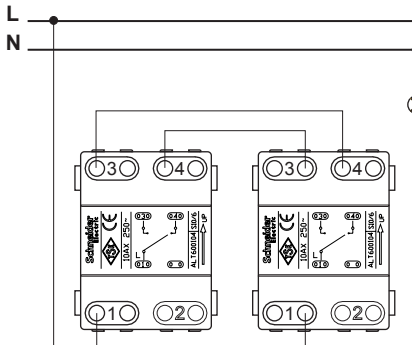
Управление одной нагрузкой с двух мест
